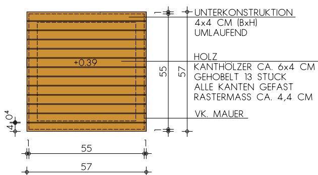
DRAUFSICHT SITZQUADER M1:10
