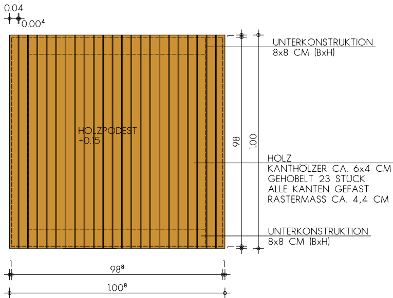
DRAUFSICHT HOLZPODEST M1:10
