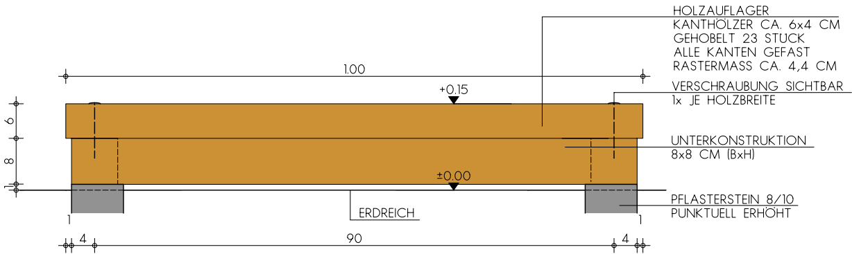
DETAIL: ANSICHT STIRNSEITE HOLZPODEST M. 1:5
