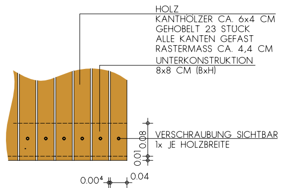
DETAIL: GRUNDRISS HOLZPODEST M. 1:5
