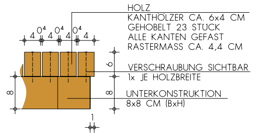
DETAIL: RAND 1:5
