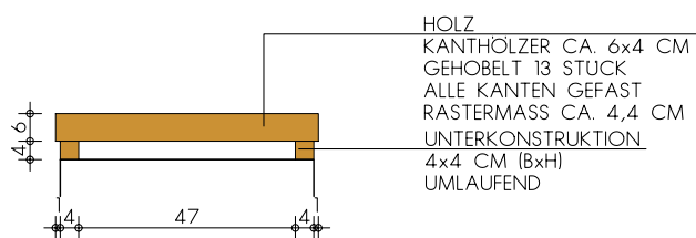
SCHNITT SITZQUADER M1:10
